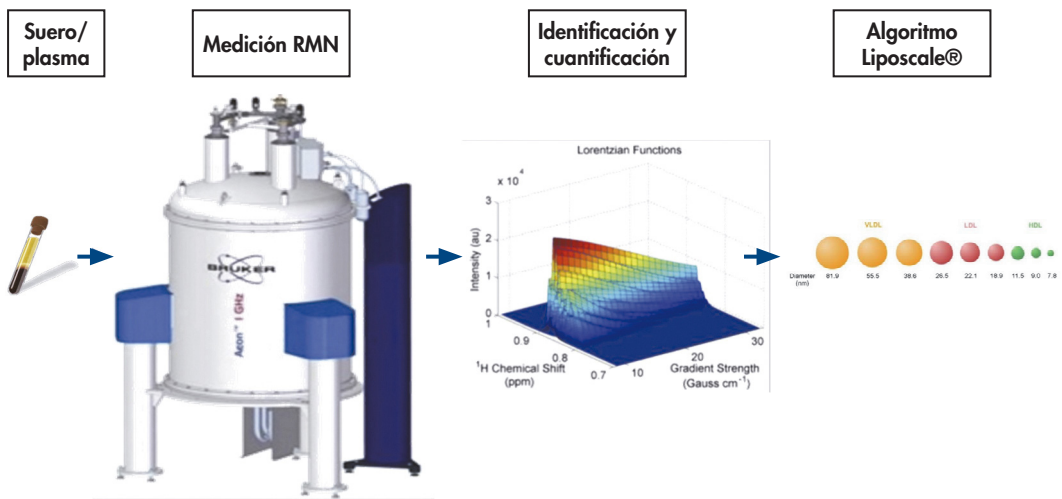
Figura 1. Procedimiento Liposcale®. Cuando se analiza una muestra de suero o plasma, se obtiene el espectro de resonancia (contiene las resonancias de cada una de las partes de cada una de las moléculas que contiene la muestra) que permite identificar y cuantificar la concentración de moléculas, pues la concentración de una determinada molécula es directamente proporcional al número de grupos que resuenan a una determinada frecuencia. La señal más utilizada para cuantificar lipoproteínas es la señal asociada a los grupos metilo debido a una particularidad de la respuesta de estos grupos de los lípidos cuando viajan dentro de las lipoproteínas 34-36 .
